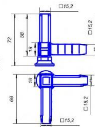
Коннектор 3 с регулируемой опорой
