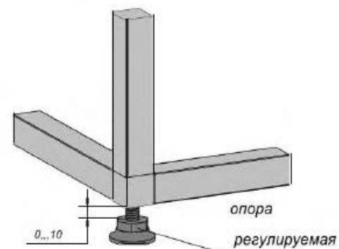
4. С использованием регулируемой опоры (регулирование по высоте 0...10мм )
