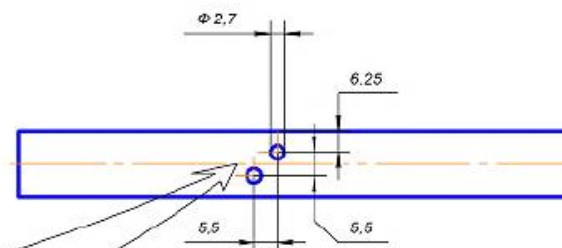
Разметка отверстий для крепления коннектора 1
