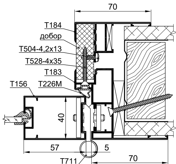
Полотно из профиля T156
