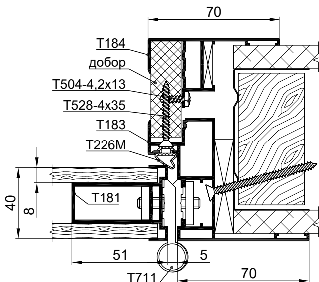
Полотно из профиля T181 (серия "LUX")
