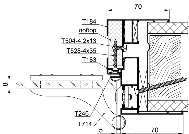
Цельностеклянное полотно толщиной 10 мм
