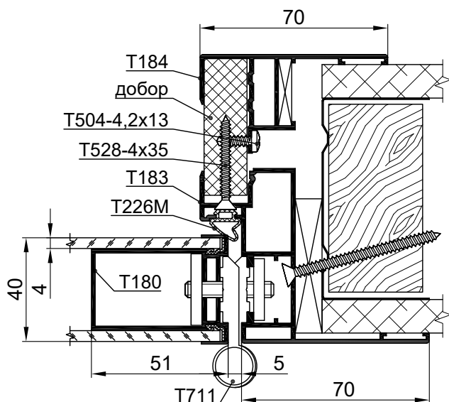
Полотно из профиля T180 (серия "LUX")
