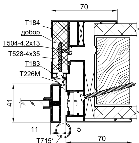
Полотно серии "Premium 1"
