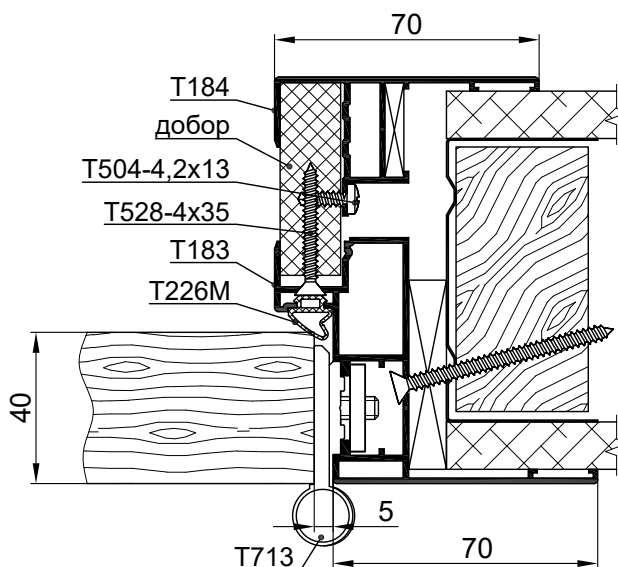
Деревянное полотно толщиной 40 мм
