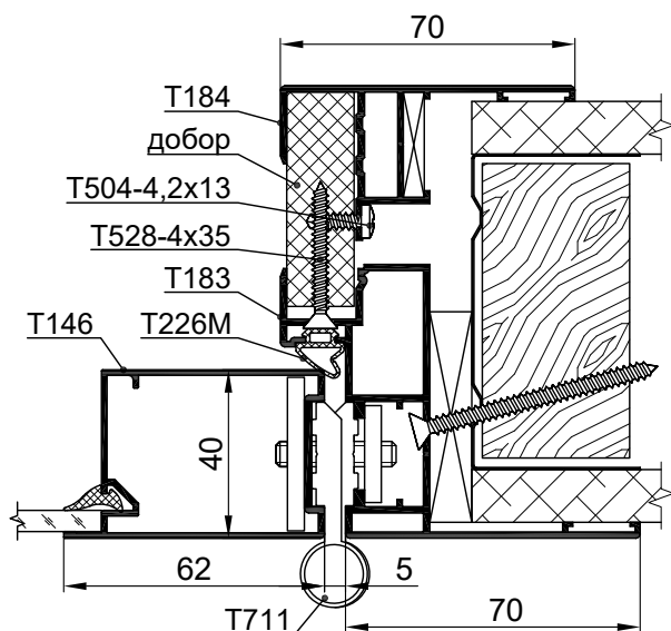
Полотно из профиля T146
