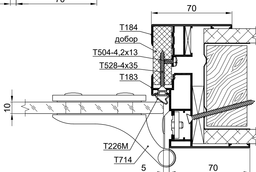
Цельностеклянное полотно толщиной 10 мм
