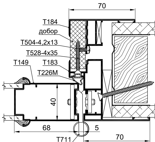
Полотно из профиля T149
