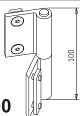
Петля дверная левая, 100 мм
